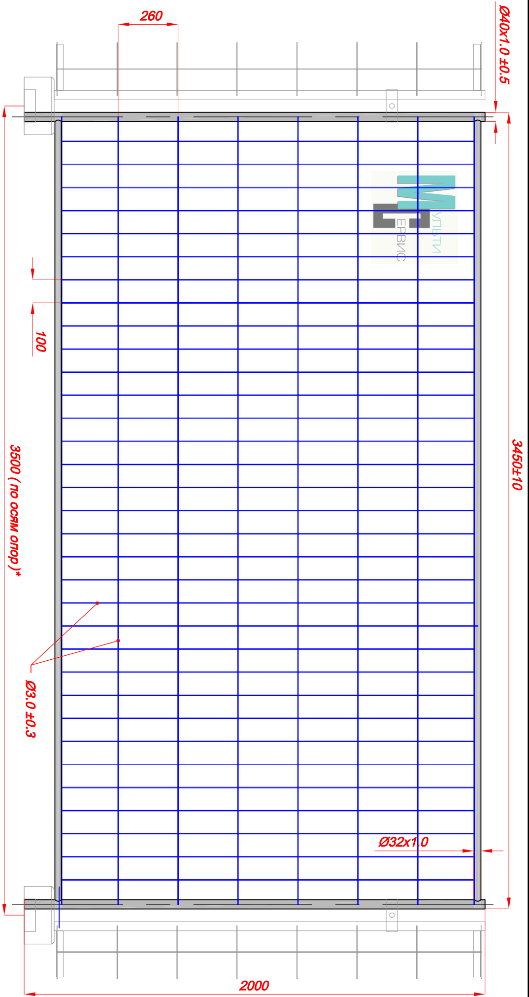
Сварка по 1/2 периметра
